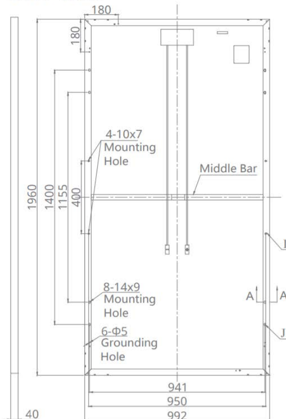
Ilustración 9. Cotas del panel fotovoltaico
