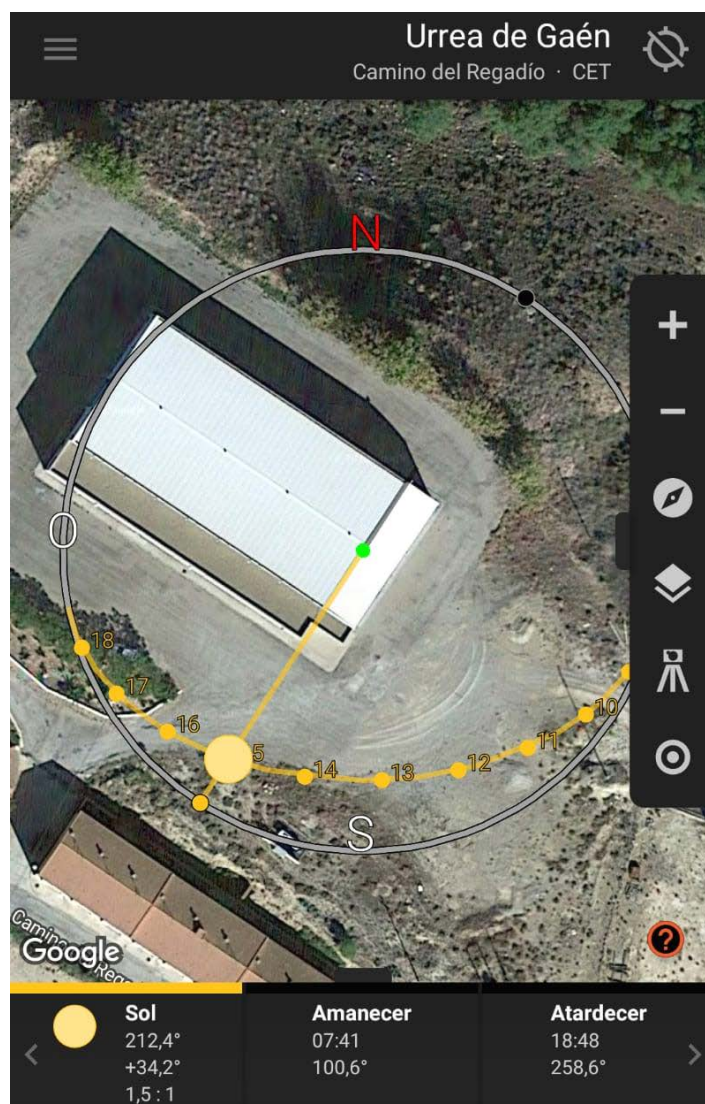
Ilustración 5. Orientación de la cubierta
