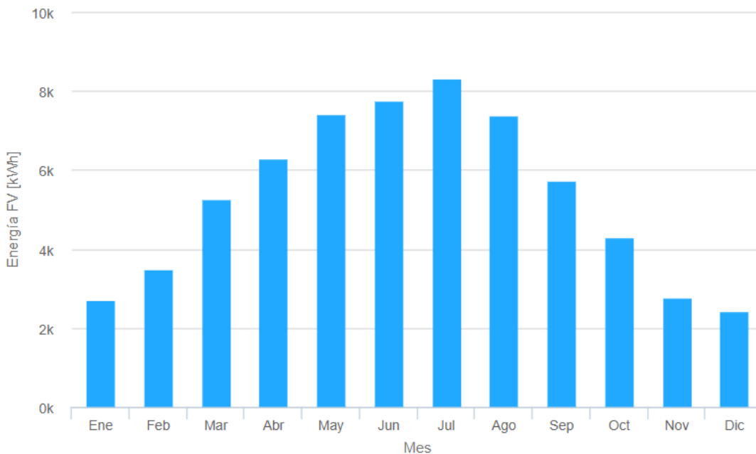
Ilustración 8. Producción anual fotovoltaica
