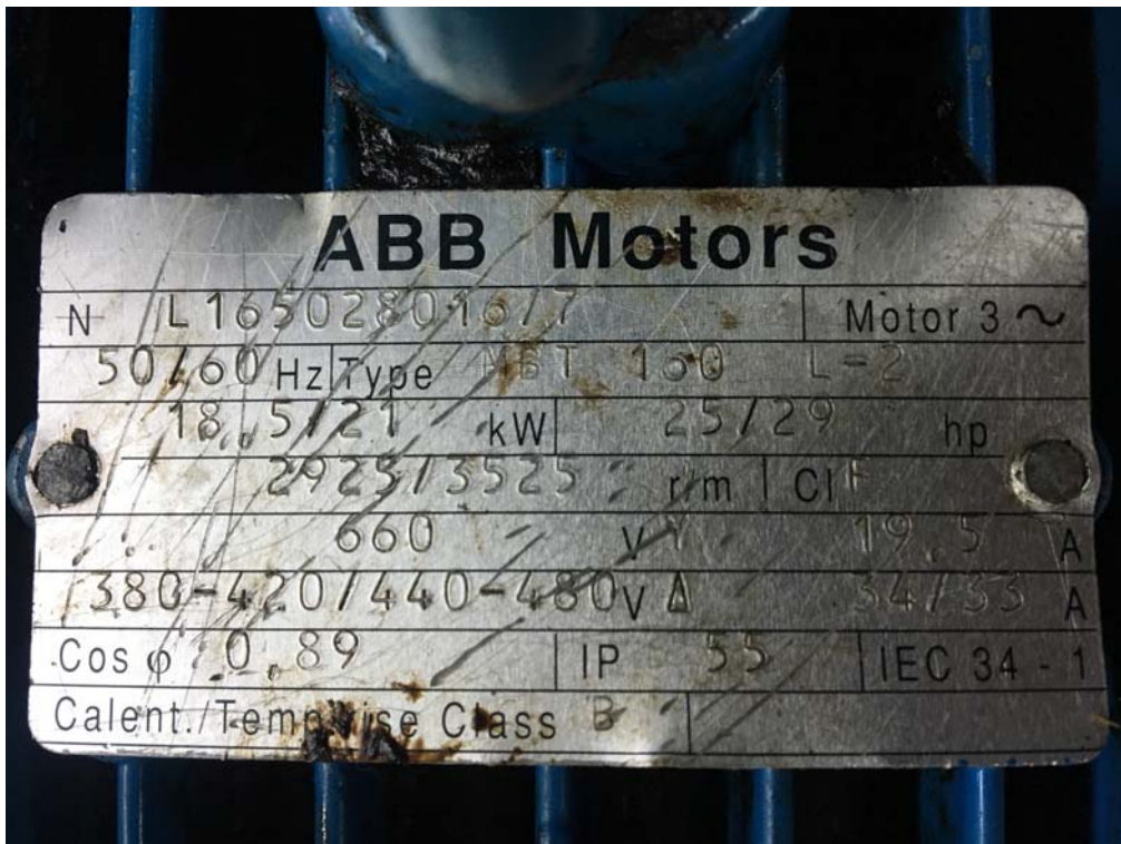
Ilustración 12. Detalle de la placa de características de motor
